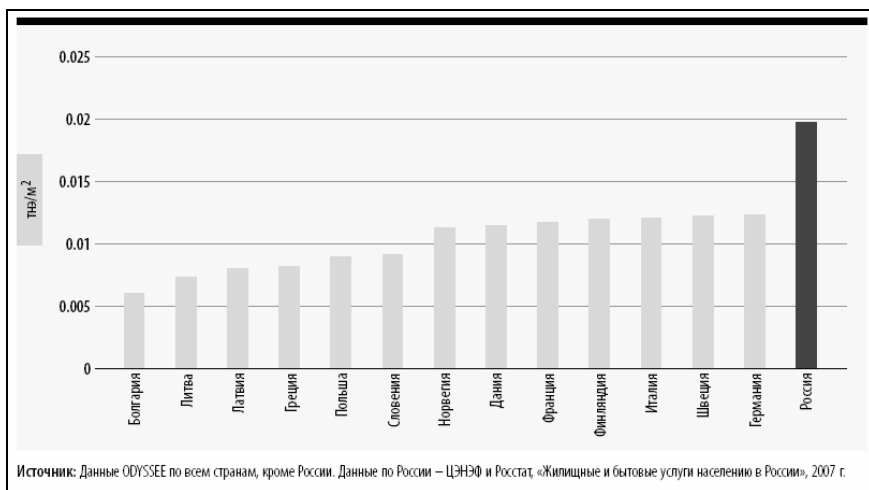
Рис. 2. Сравнение показателей энергоэффективности систем отопления жилых зданий (2004 г.)
