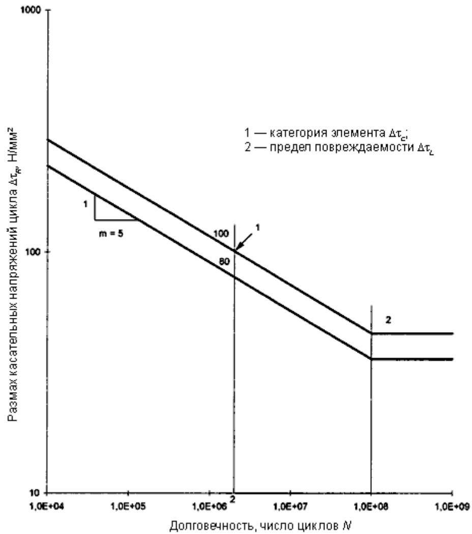
Рисунок 7.2 — Кривые сопротивления усталости для размаха касательных напряжений цикла
